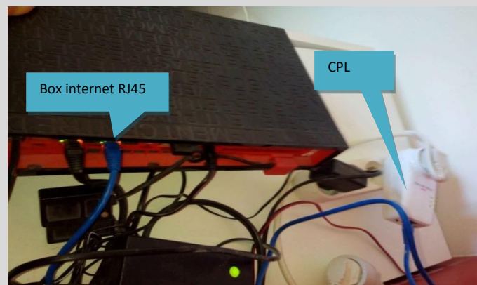
1 Brancher le câble Ethernet coté Box et CPL
