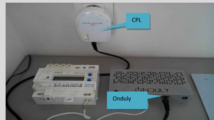
3 Brancher le connecteur RJ45 au CPL et à l'Onduly
